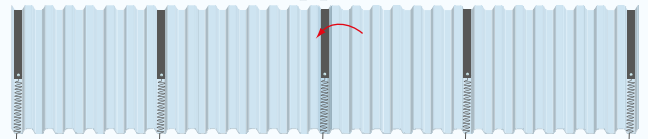
Montage par sangle pour capots n° 5 et plus grands
