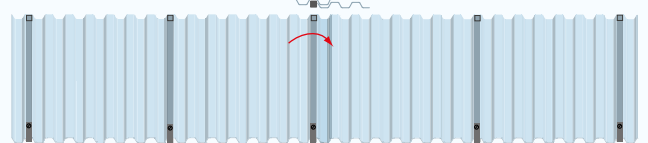
Montage par sangle pour capots n° 5 et plus grands
