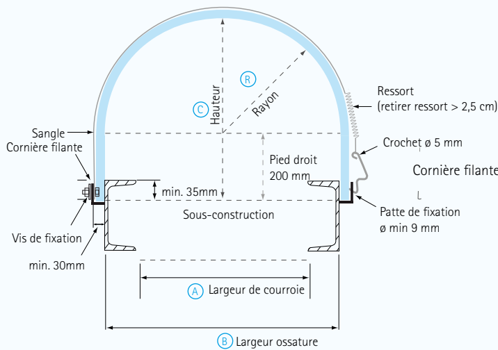
Montage par sangle pour capots n° 1 - 2 - 3 - 4
