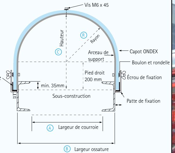
Montage par sangle pour capots n° 5 et plus grands
