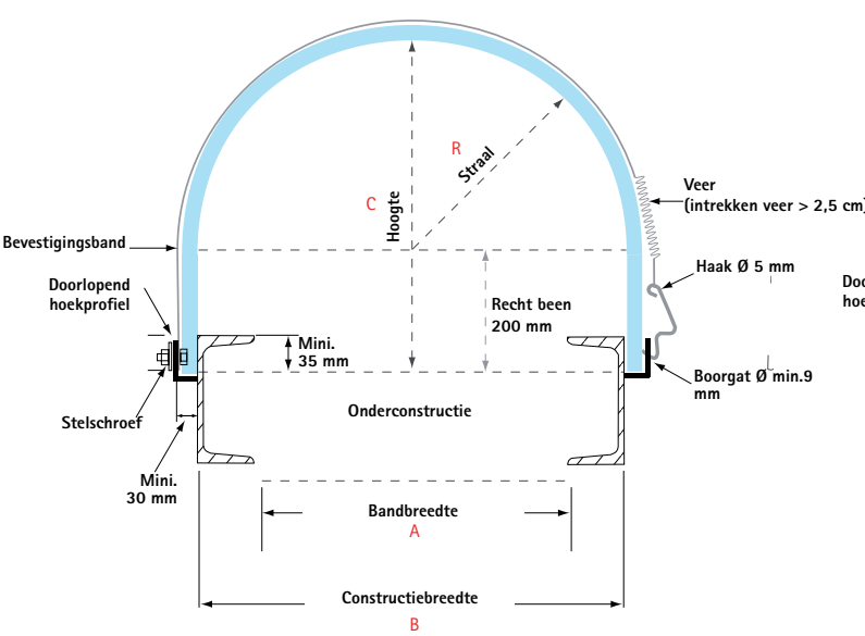
Bevestiging met bevestigingsbanden voor kap n° 1-2-3-4
