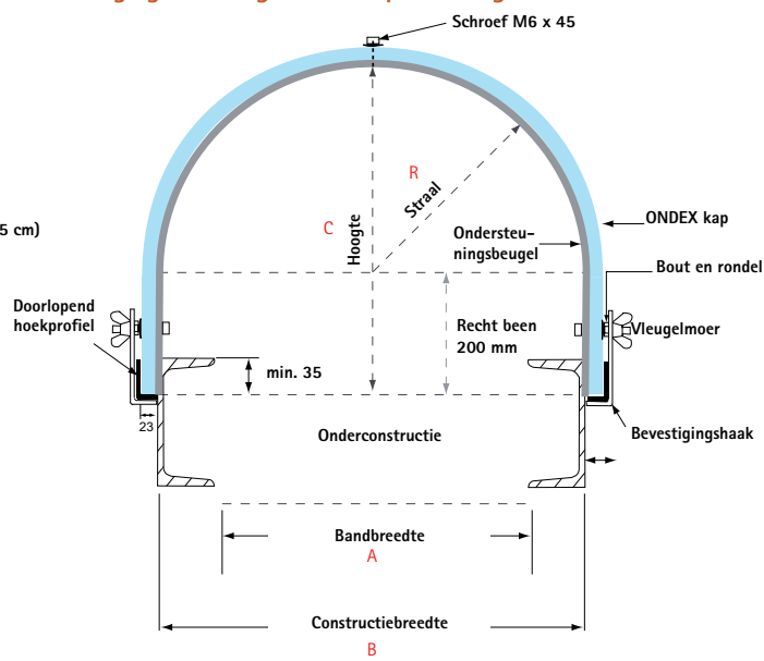
Bevestiging met beugels voor kap n° 5 en groter
